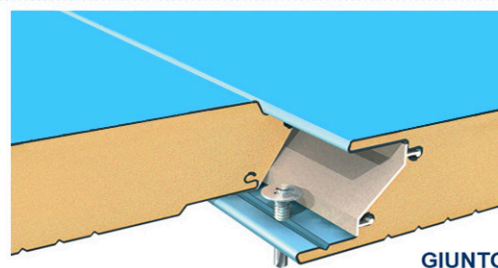
GIUNTO
